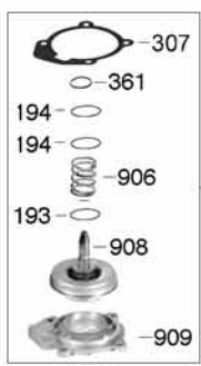
Servo
